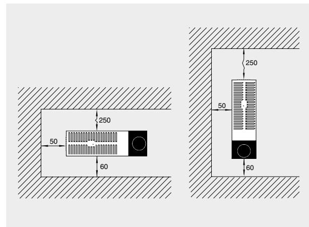
Fig. 1: Minimimått vid fast montering.
